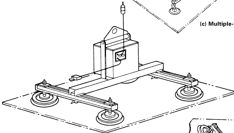
(d) Four-Pad Powered Vacuum Lifter
